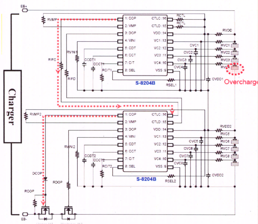
图2 锂离子电池过充电时的保护电路工作原理图
