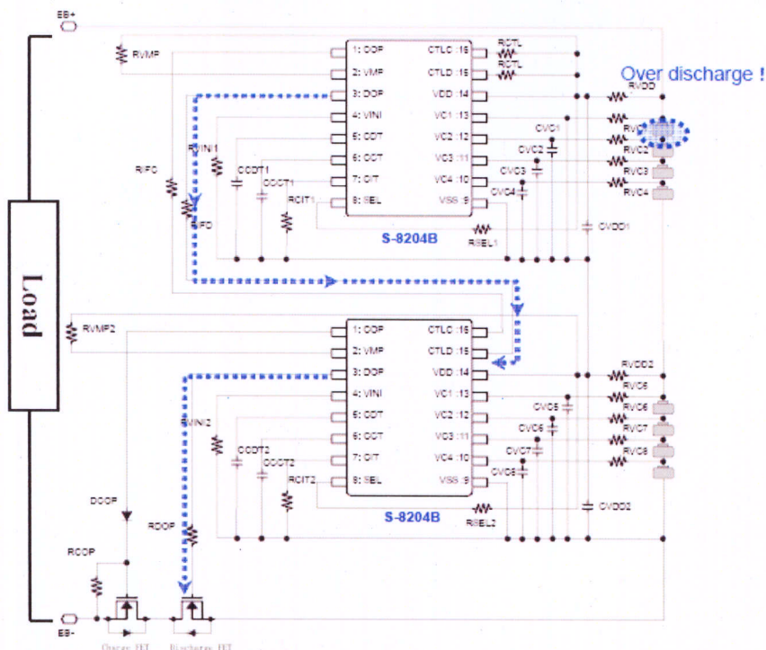
图3 锂离子电池过放电时的保护电路工作原理图
